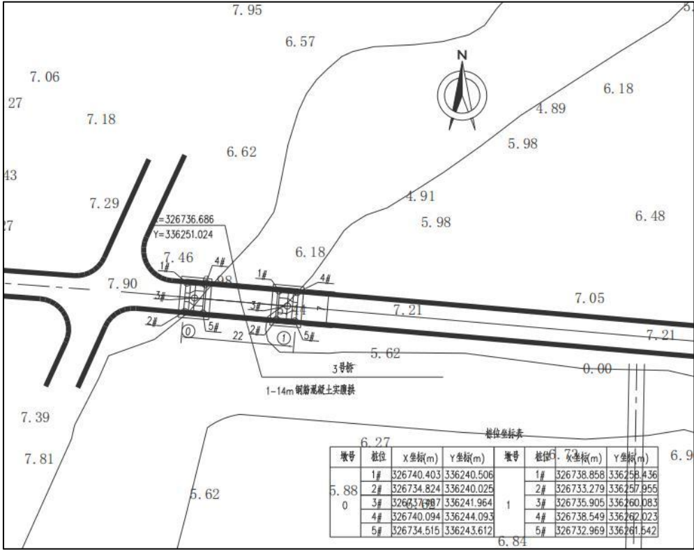
图3.7-6 3#桥梁平面图
