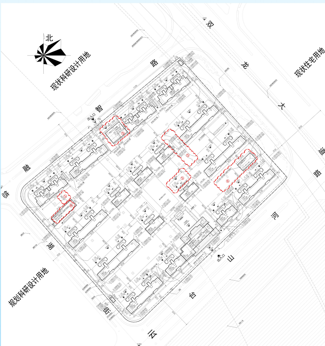
调整后总平面图
