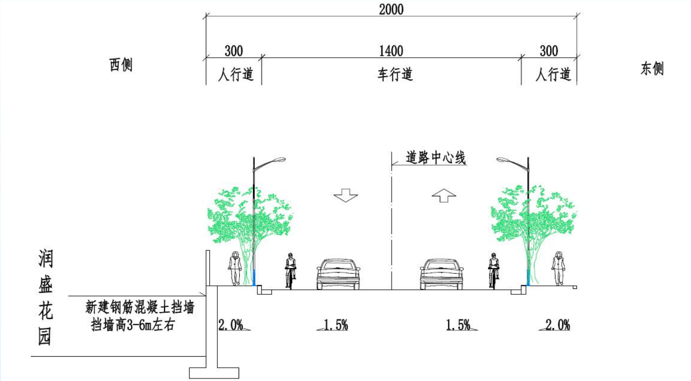
支13路（润盛花园段）横断面图
