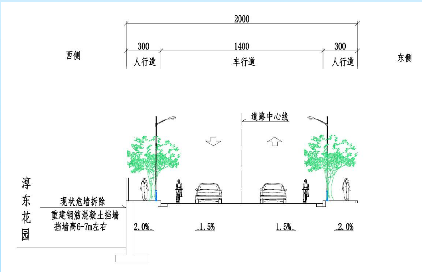
支 13 路（淳东花园段）断面图
