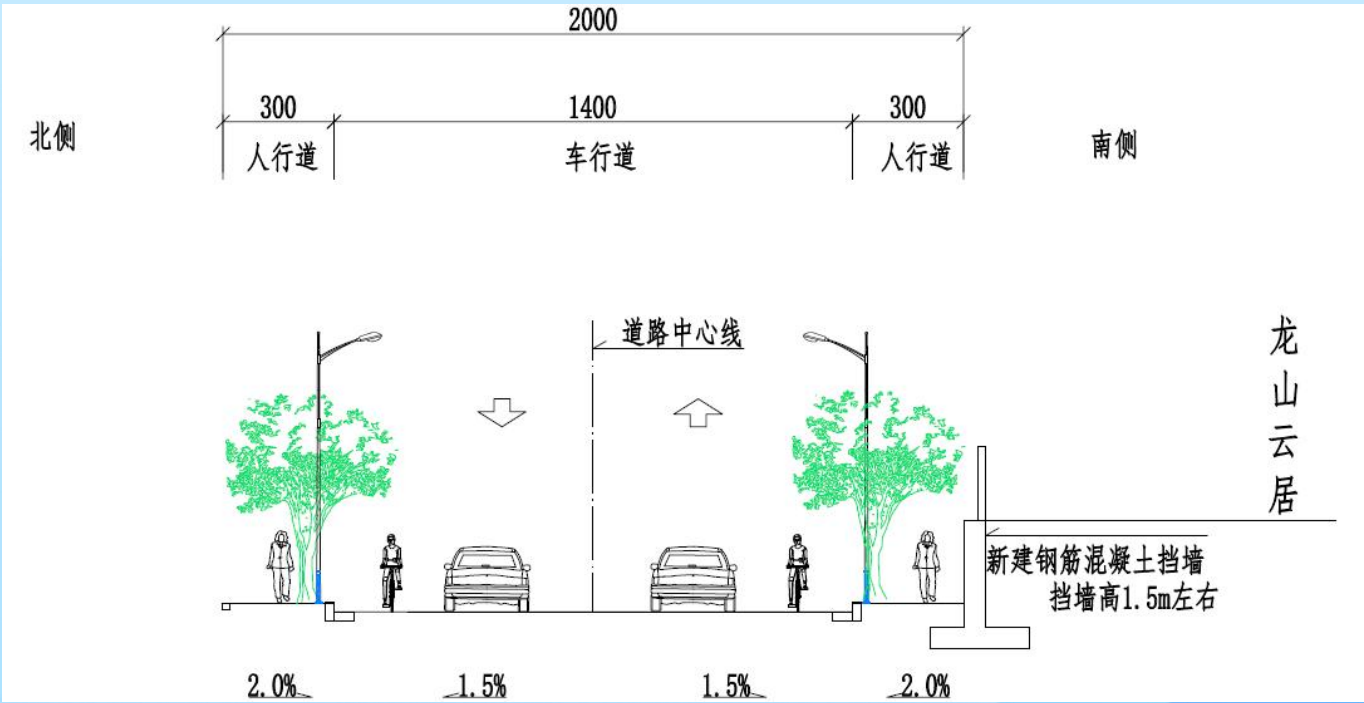
支15路（龙山云居段）横断面图
