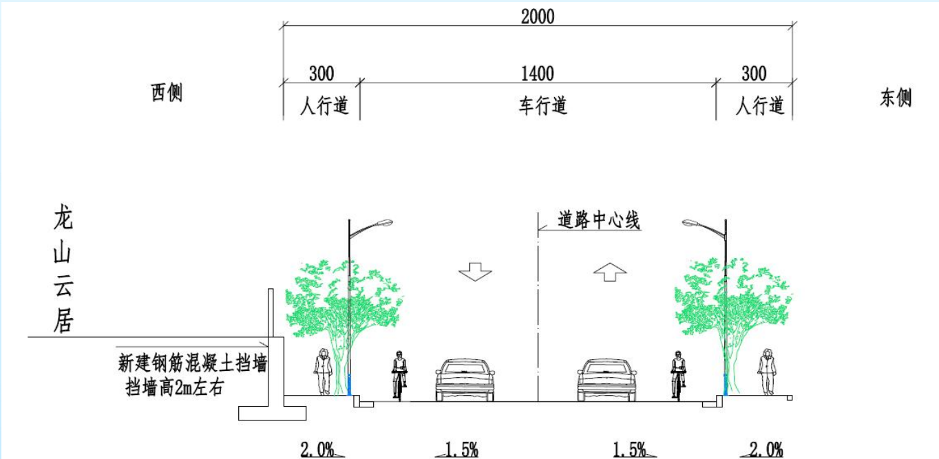
支14路横断面图
